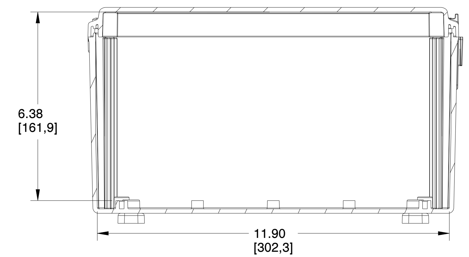
SECTION A-A
