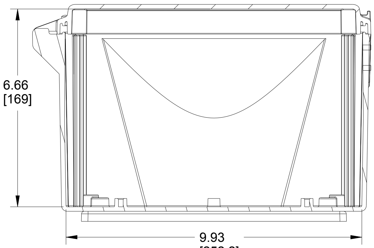
SECTION A-A
