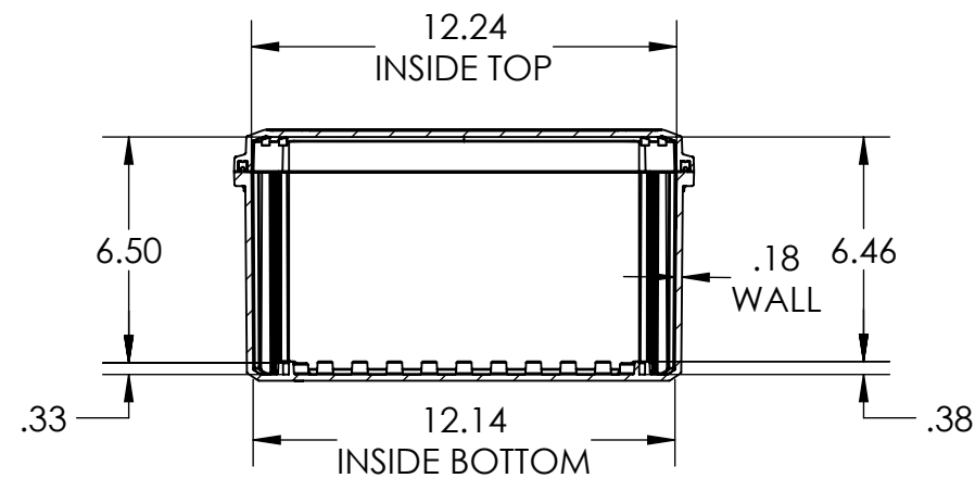
SECTION A-A SCALE 1 : 6
