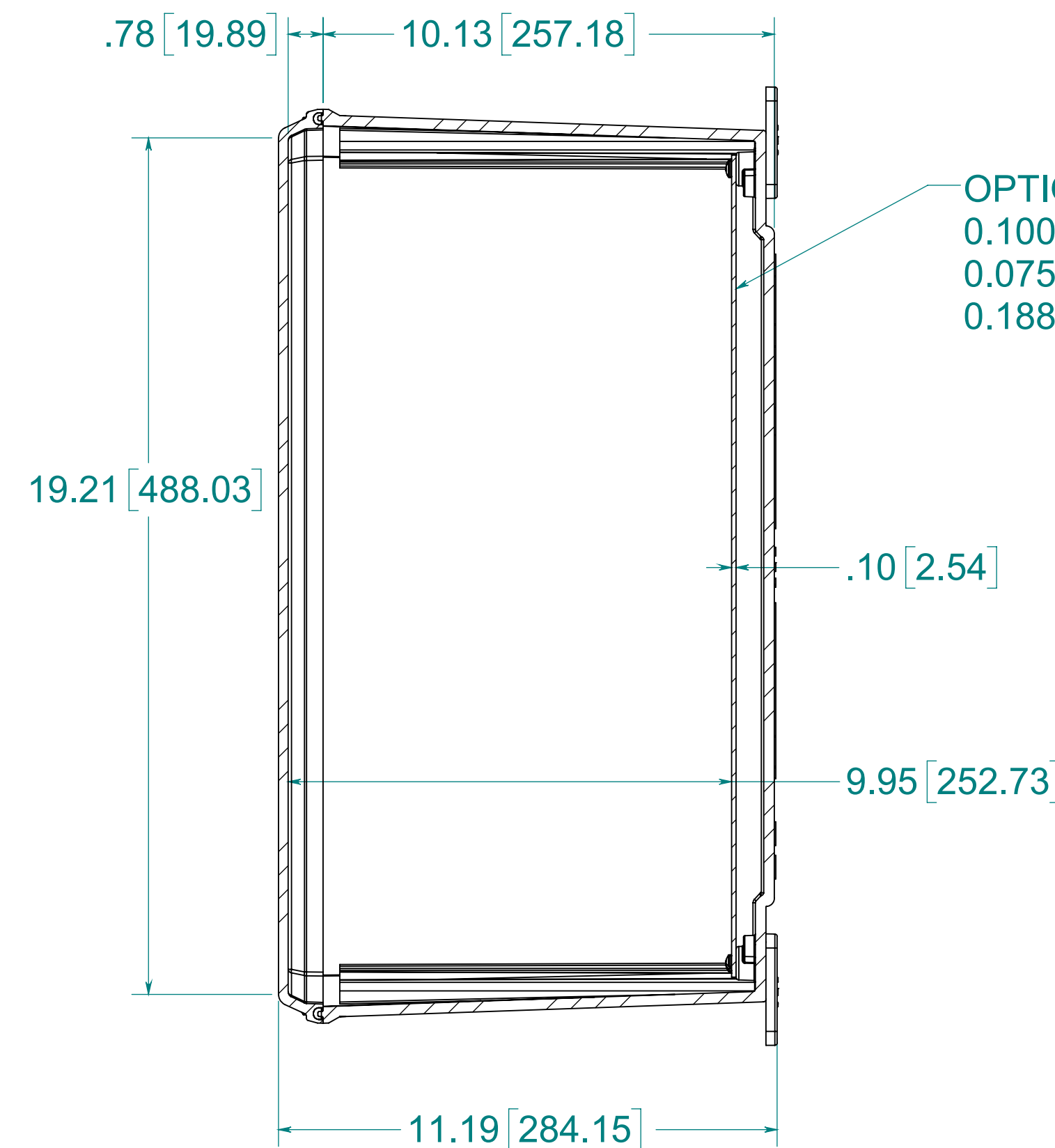
SECTION A-A
